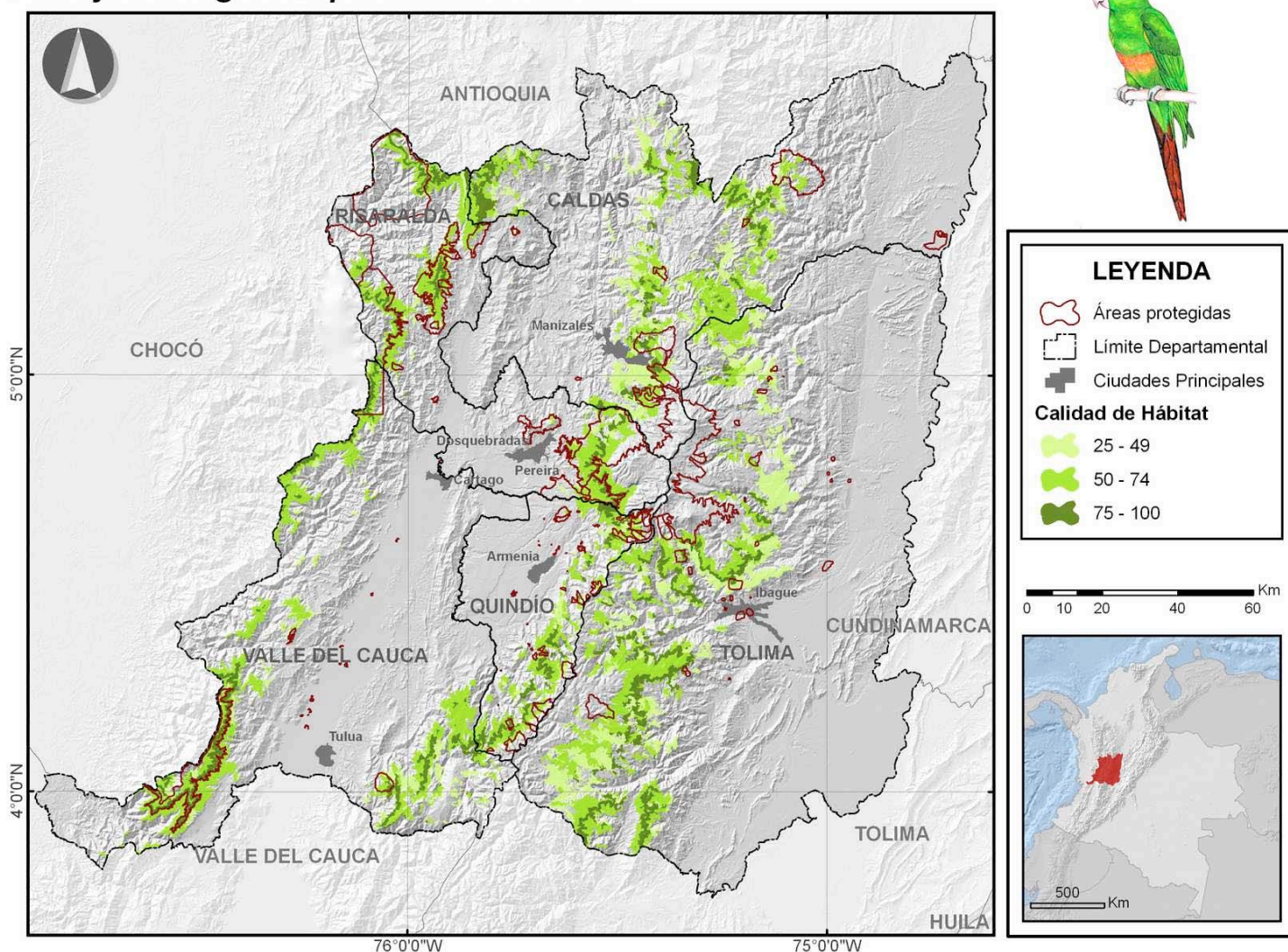
Figura 3. Modelo de distribución potencial del Perico paramuno para la región del SIRAP-EC. Los colores corresponden a las probabilidades de ocurrencia de la especie en la región.
